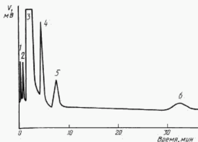
Типовая хроматограмма этиленгликоля с использованием колонки II
