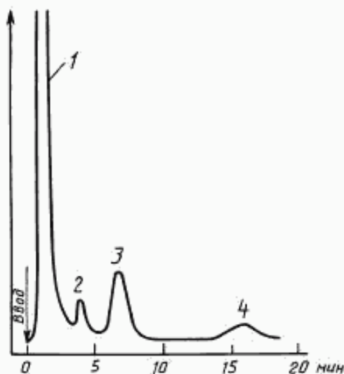
Типовая хроматограмма этиленгликоля с использованием колонки I
